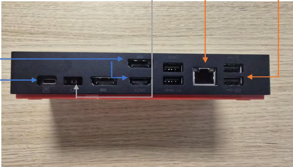
Connectiques du dock LENOVO
